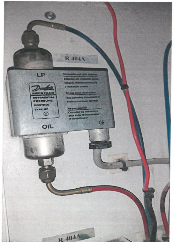
YAĞ BASINÇ KONTROL OTOMOTİĞİ (Switch)
